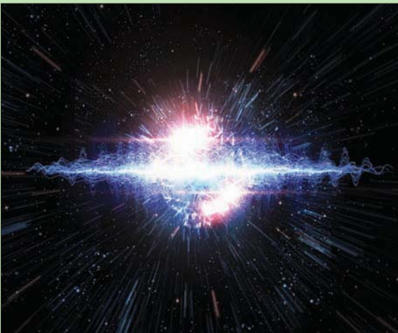
رصد أسرع انفجار نجمي (شاترستوك)
