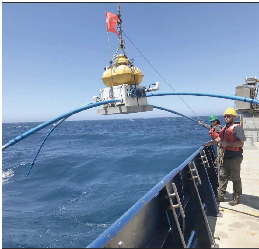
جهاز استشعار كهرومغناطيسي في طريقة للقاء لجمع البيانات (الفريق البحثي)
