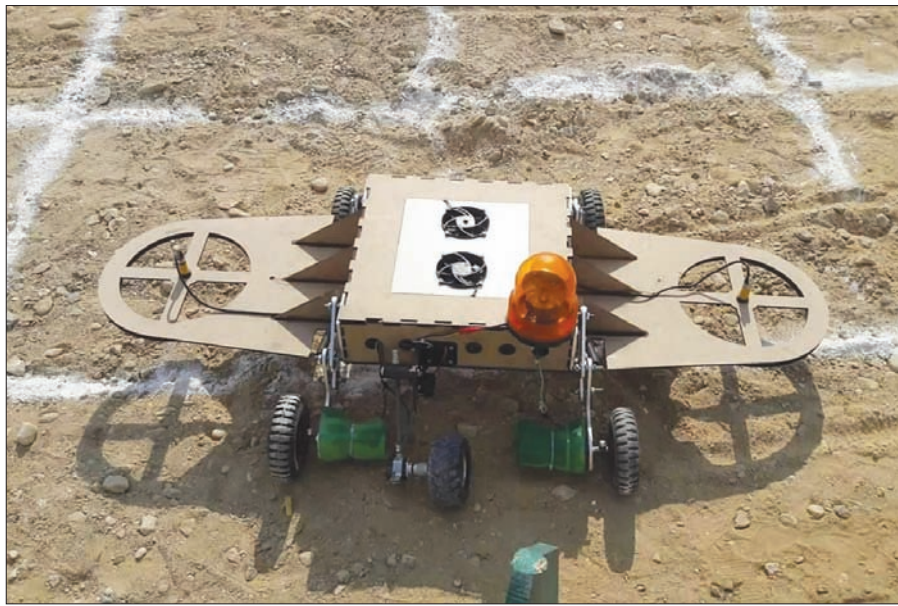
روبوت الكشف عن الأنغام الذي ابتكره طلاب كلية الهندسة بجامعة بنها
